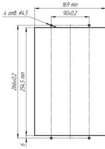
а) БЭ2704 1XX
