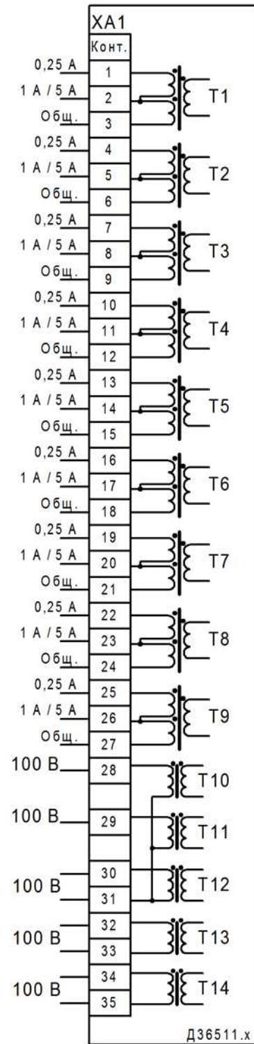
е) конфигурация 9ТТ и 5ТН
