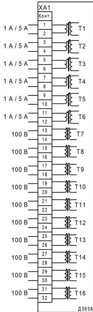
а) конфигурация 6ТТ и 10ТН
