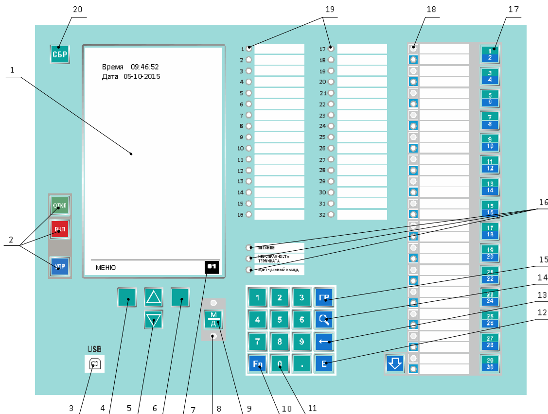
в) терминал БЭ2704 312
