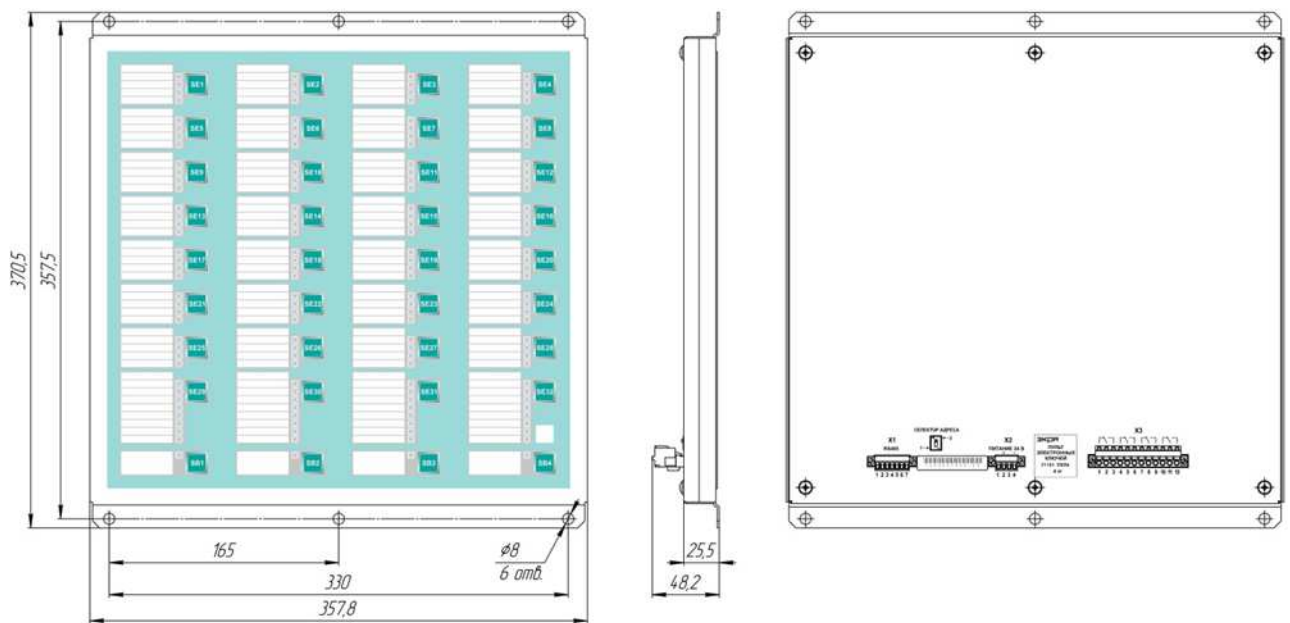
Рисунок Ж.10 – Общий вид и габаритные размеры пульта электронных ключей У1181
