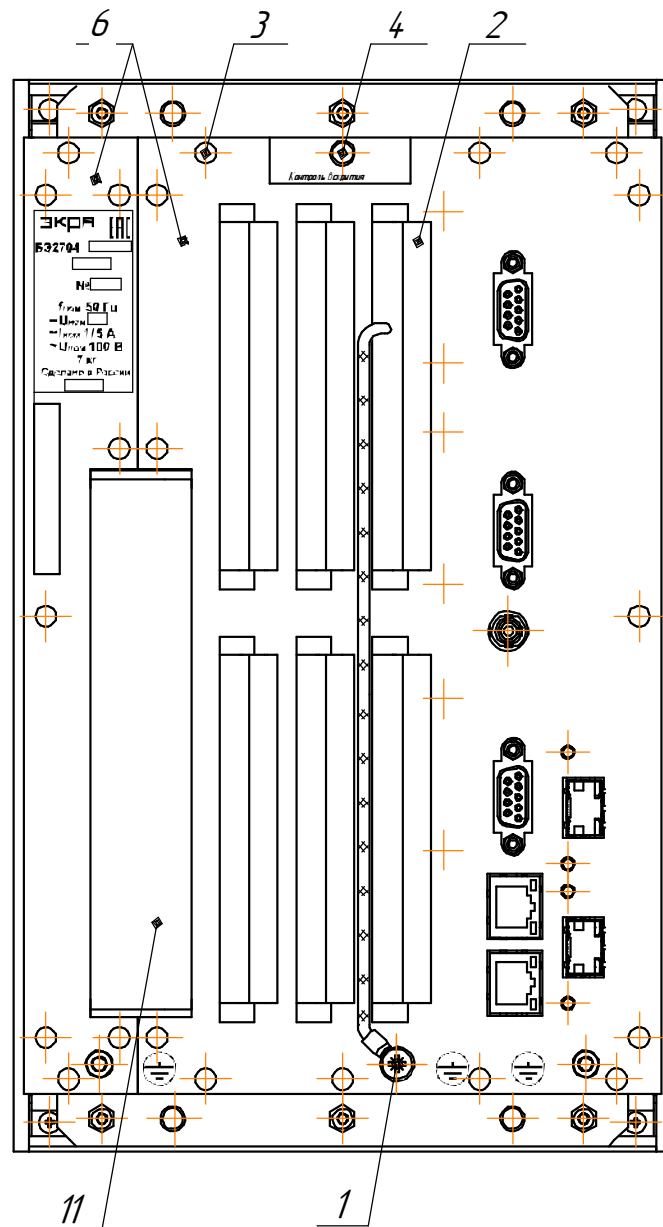
д) вид сзади аппаратов 102 и 103
