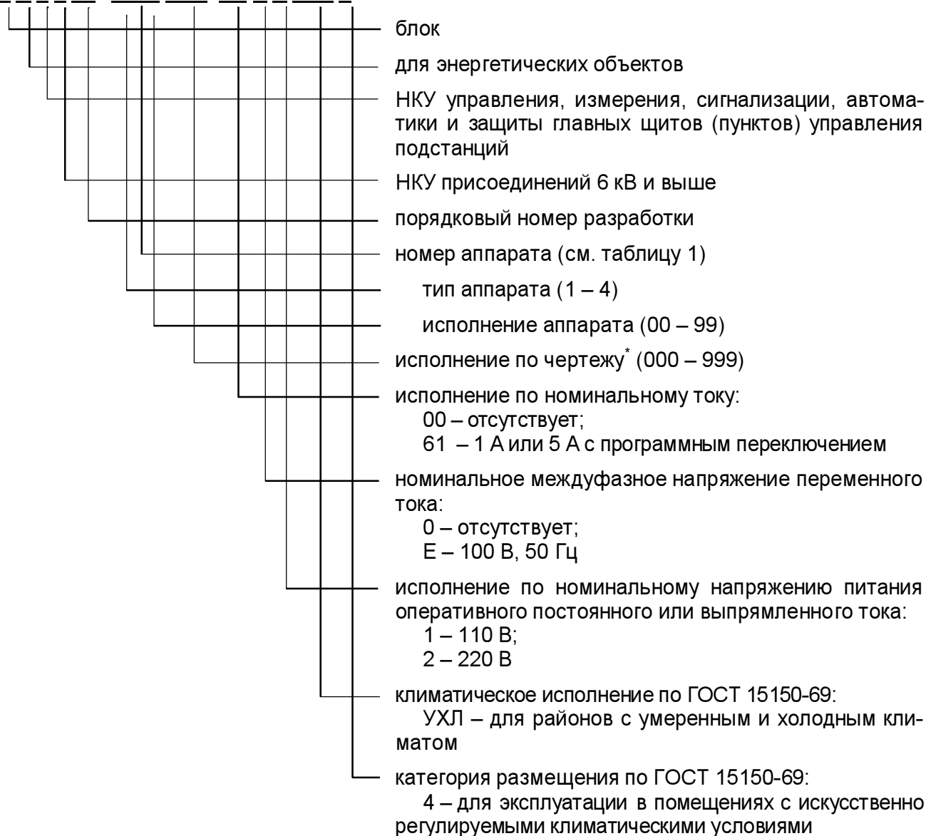
Т а б л и ц а 1 – Аппаратное исполнение терминалов
