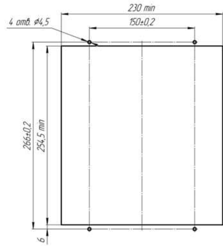
б) БЭ2704 2XX
